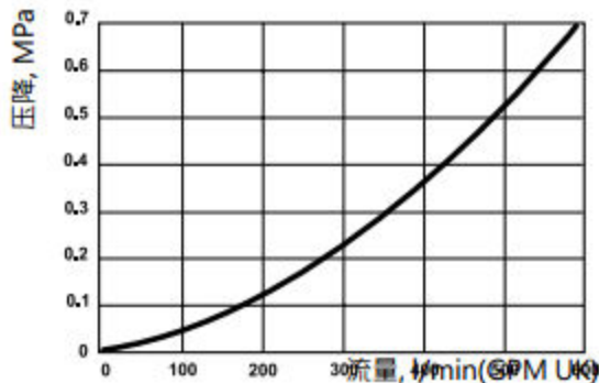
压降图
