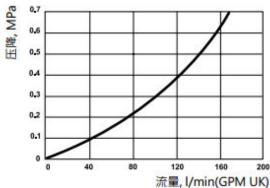
压降图
