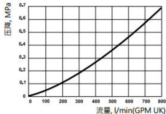
压降图
