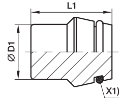
X1) O型圈
