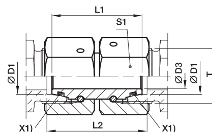
X1) O型圈
